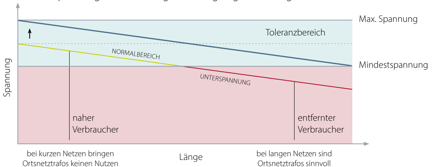
Spannungsabfall bei langen Leitungen grafisch dargestellt
